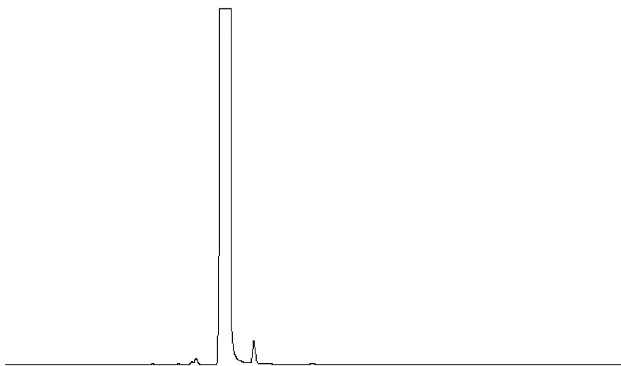
图 B.1 食品添加剂己酸乙酯气相色谱图
